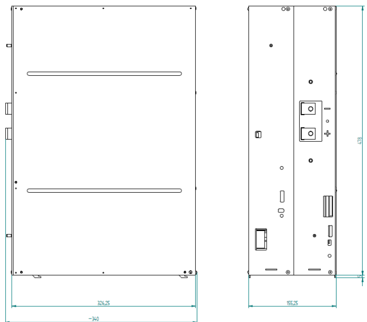
Maßskizze (mm)
